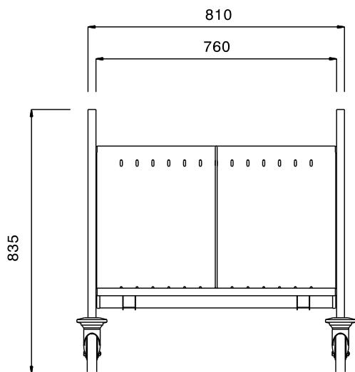
Front aanzicht
